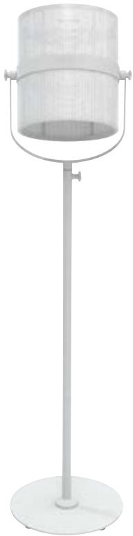
ラ・ランプバリ／ホワイト＋ホワイト La Lampe Paris/White+White 照明外径／W287×D250×H361mm ベーススタンド／φ350×H1,684mm 主材／アルミ、OTF 重量／13.5kg 組立式 ¥110,000(本体価格 ¥100,000)
